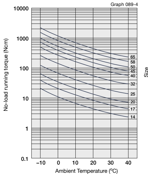
Input speed: 3500rpm
