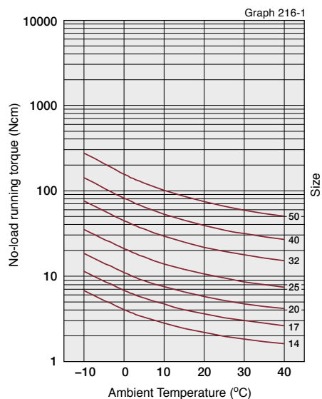
Input speed: 500rpm
