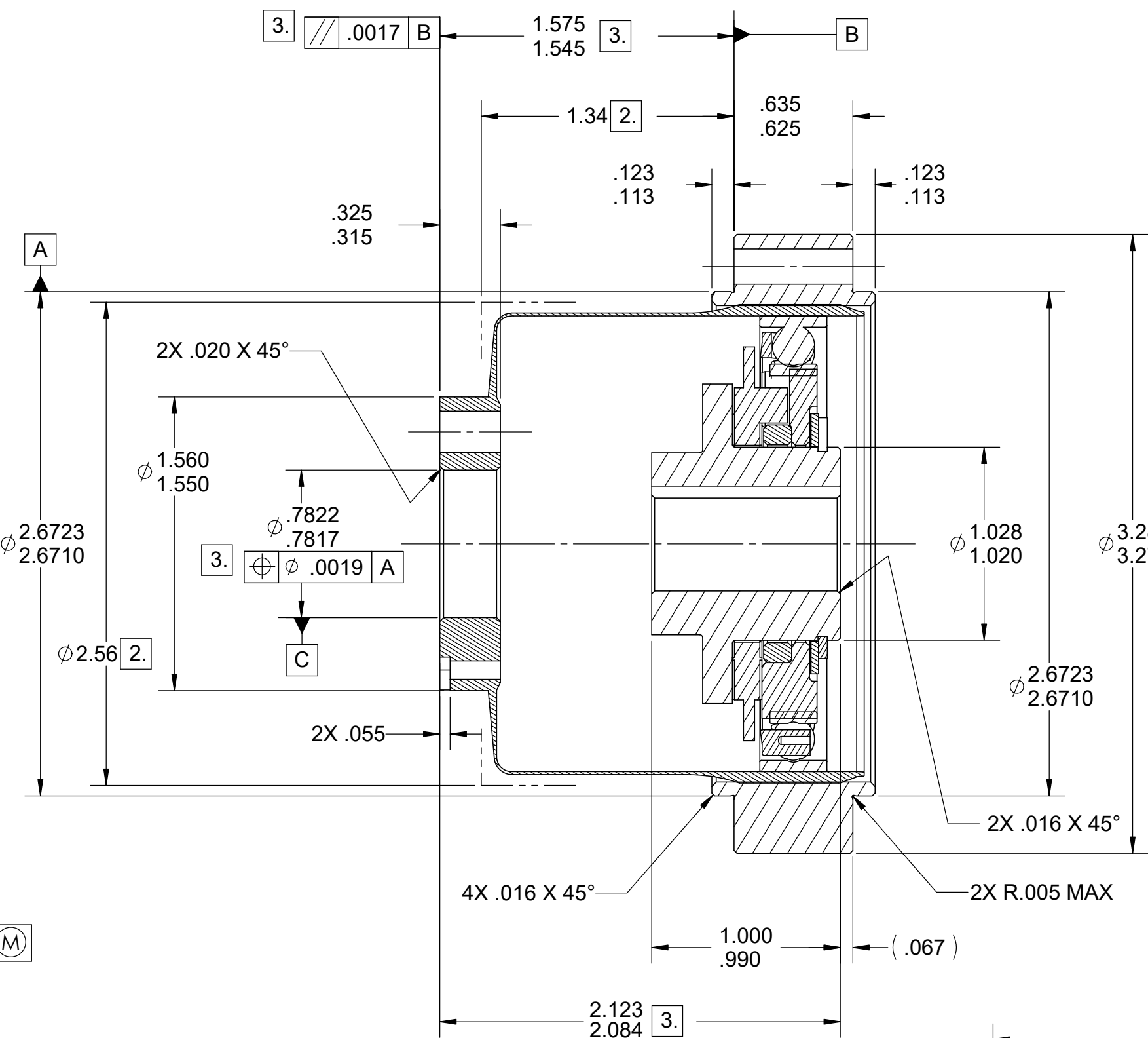
SECTION A-A
