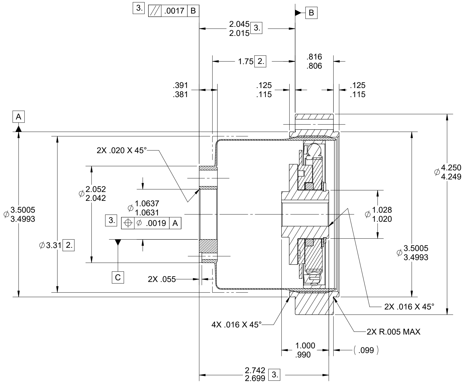
SECTION A-A
