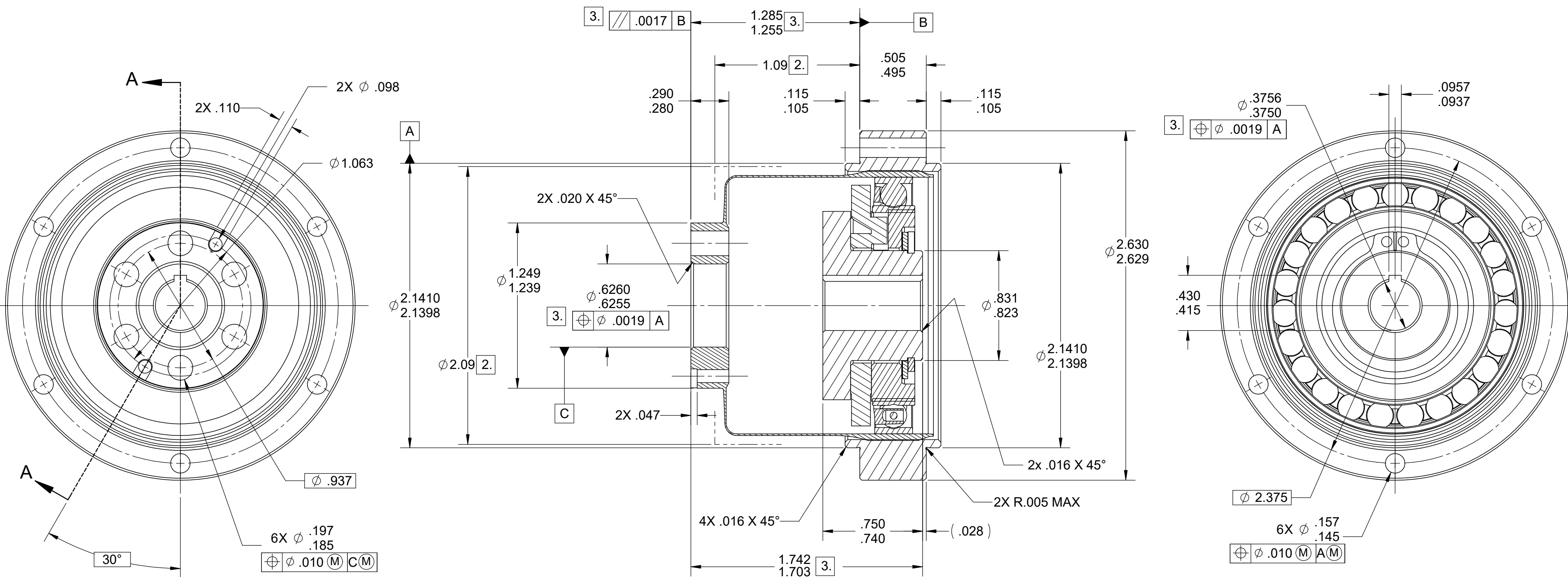
SECTION A-A
